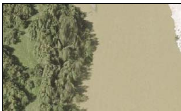
FIGURA 11. Aplicación de LiDAR en el estudio del sombreado de la vegetación riparia sobre el cauce (Fuente: elaboración propia).
