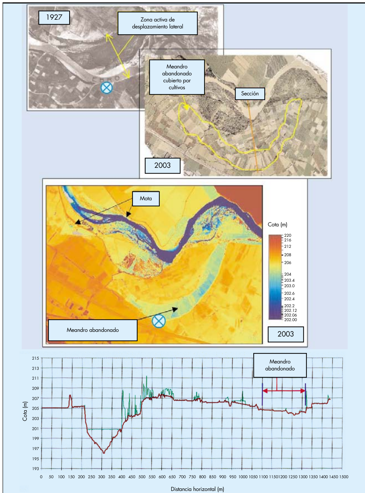
FIGURA 7. Estudio de la evolución de meandros abandonados (Fuente: elaboración propia). El rango de cotas en la figura c se encuentra representado en una escala logarítmica.
